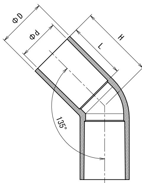
断面 A-A
